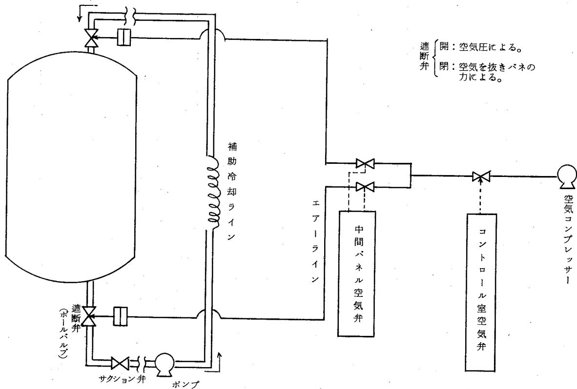
重合器補助冷却配管遮断弁の作動機構
