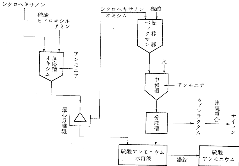
ナイロン製造中の副生硫酸アンモニウムのフローシート
