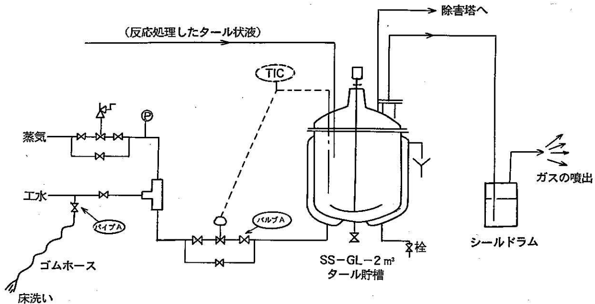
タール貯槽関係フロー
